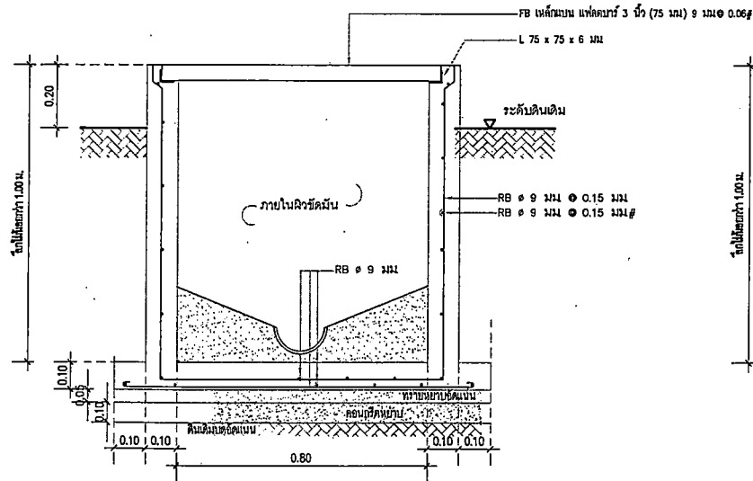
รูปตัด A ฝาปิด MANHOLE (น้ำทิ้ง)
