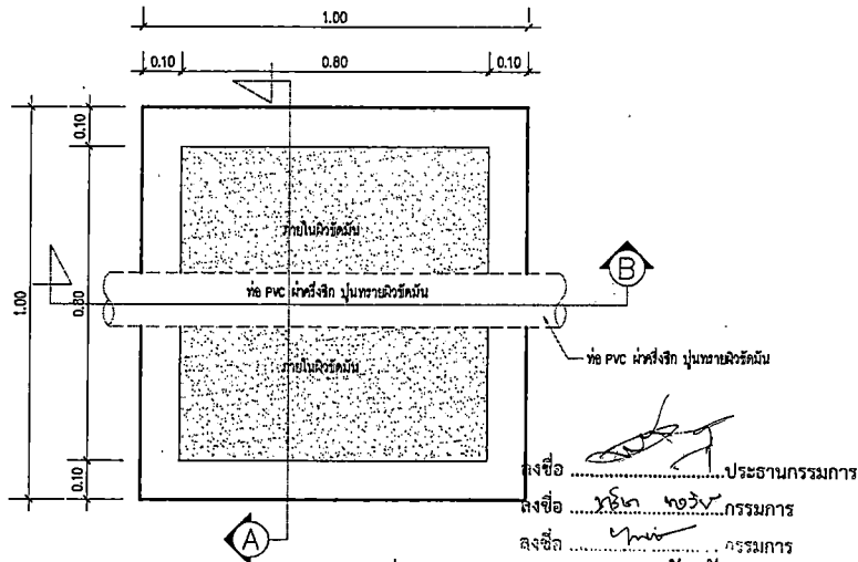
แบบขยายฝาปิด MANHOLE (น้ำทิ้ง)
