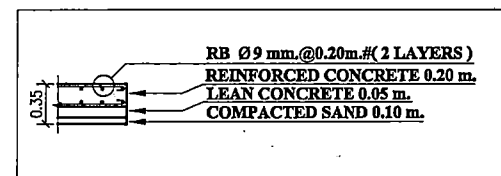
แบบขยายการยึดถึงบ่อบำบัดน้ำเสีย
