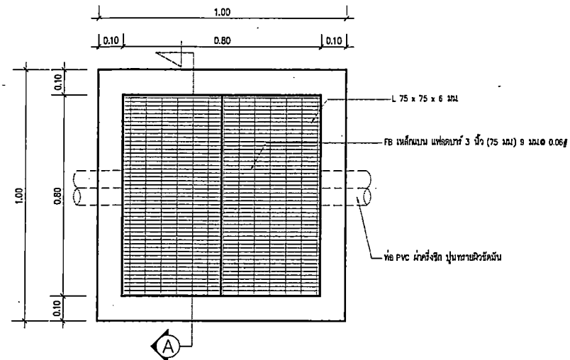
แบบขยายฝาปิด MANHOLE (น้ำทิ้ง)
