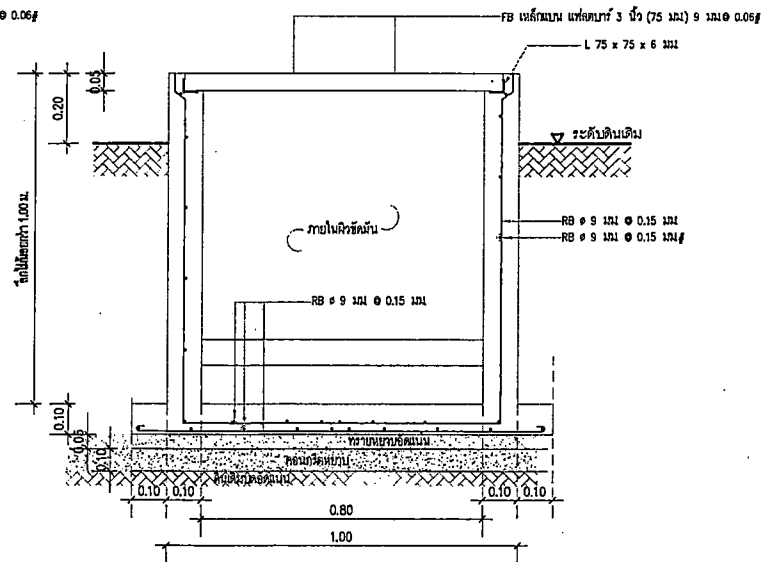
รูปตัด B ฝาปิด MANHOLE (น้ำทิ้ง)
