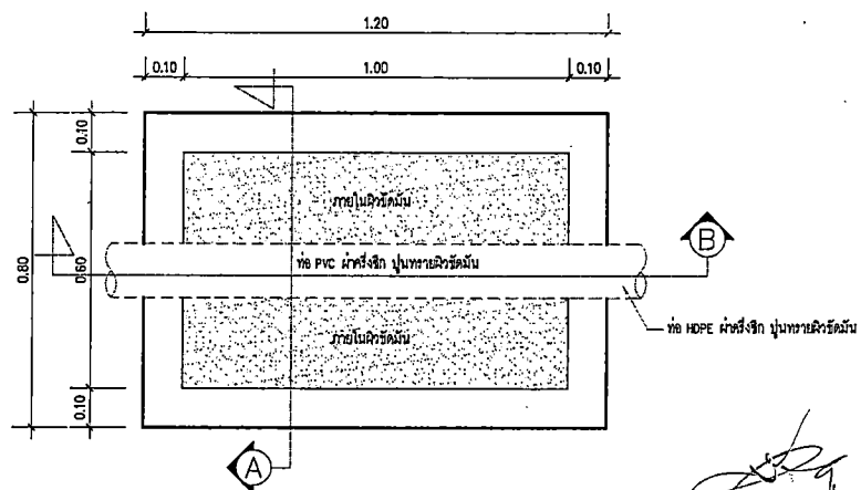
แบบขยายฝาบ่อพัก MANHOLE
