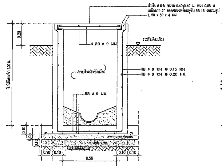
รูปตัด A บ่อพัก MANHOLE
