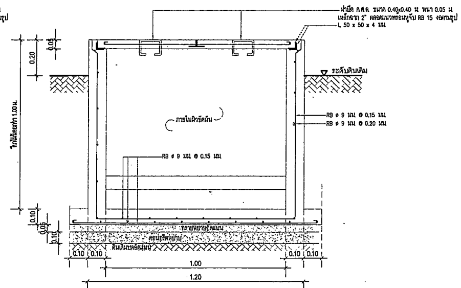
รูปตัด B บ่อพัก MANHOLE
