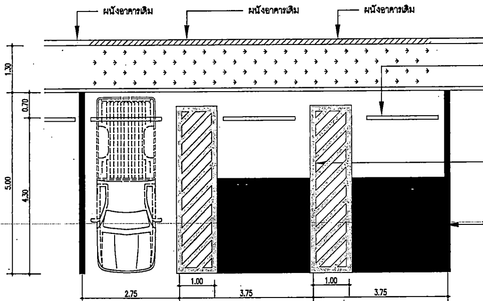
แบบขยายตีเส้นที่จอดรถคนพิการ มาตรฐาน 1:75
