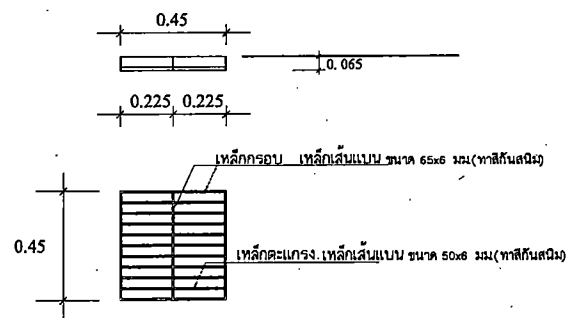
รูปตัดขยายฝาบ่อพัก 1:20
