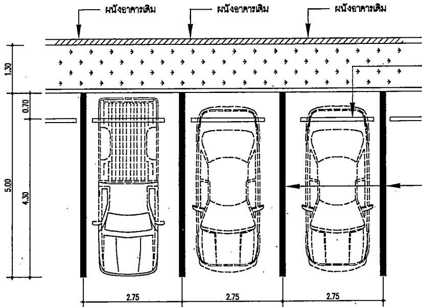
แบบขยายตีเส้นที่จอดรถยนต์ มาตรฐาน 1:75
