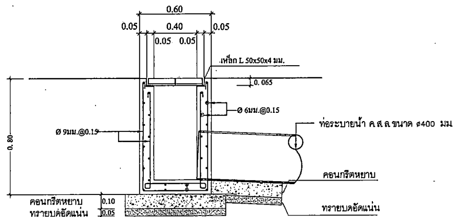
รูปตัดขยายบ่อพัก 1:20
