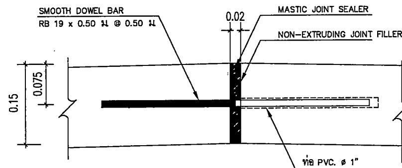
รอยต่อเพื่อการขยายตัว ( EXPANTION JOINT )
