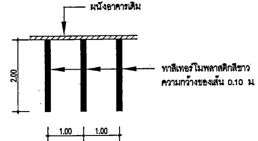
แบบขยายตีเส้นที่จอดรถมอเตอร์ไซด์ มาตรฐาน 1:75
